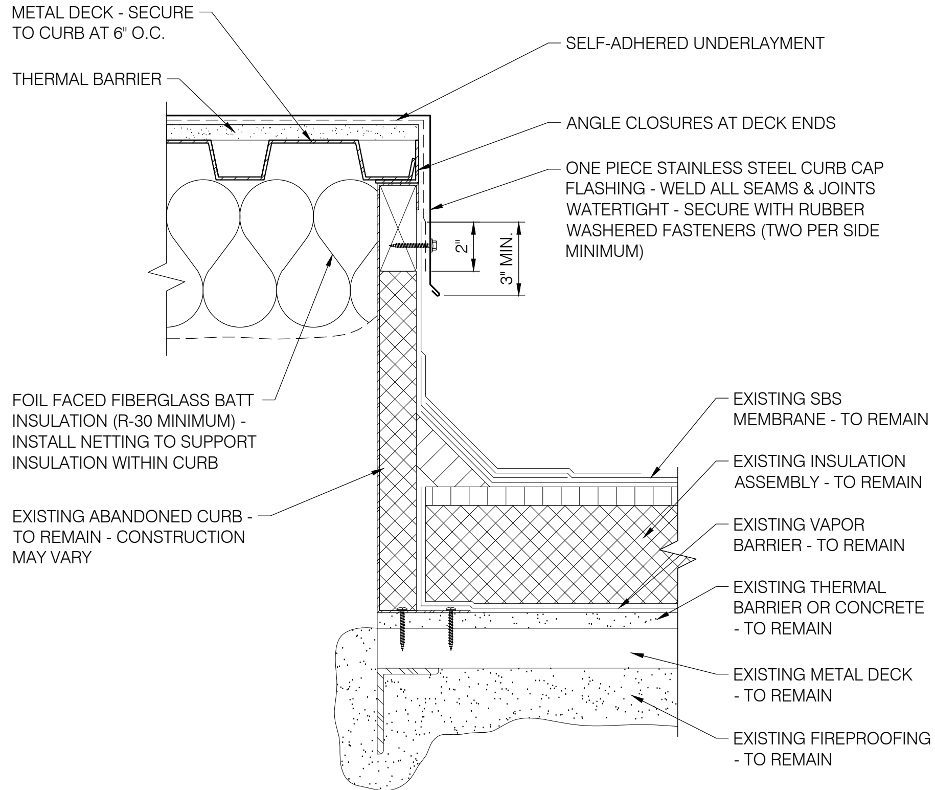
0701 SBS CURB - CAP SCALE: 3" = 1'-0"
