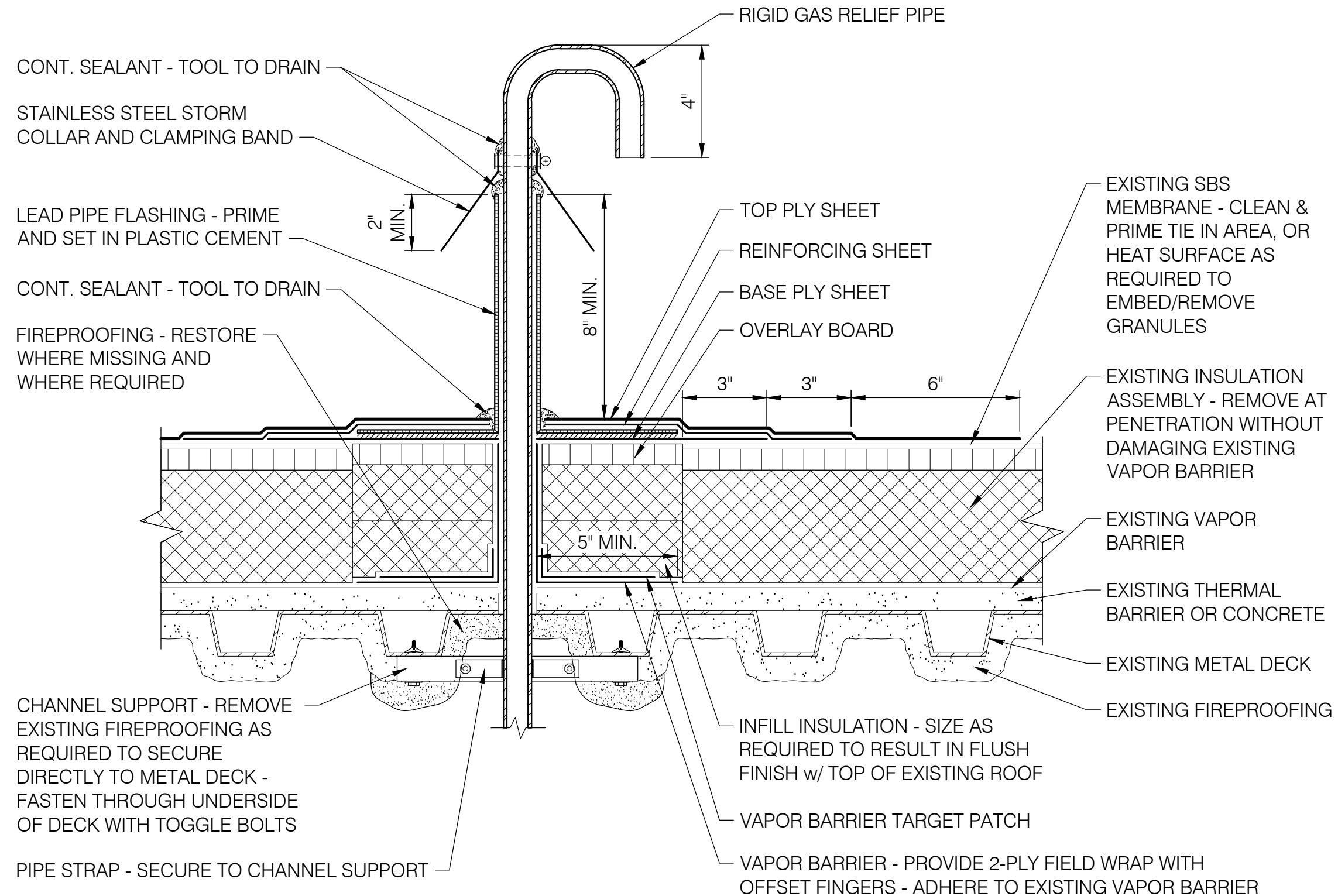
0708 SBS FLASHING - GAS RELIEF VENT SCALE: 3" = 1'-0"
