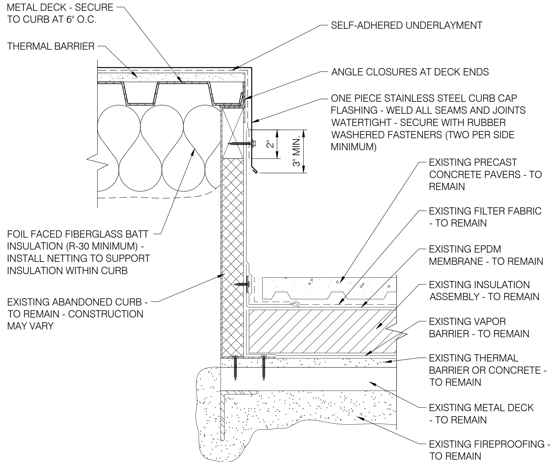
0721 EPDM CURB CAP SCALE: 3" = 1'-0"
